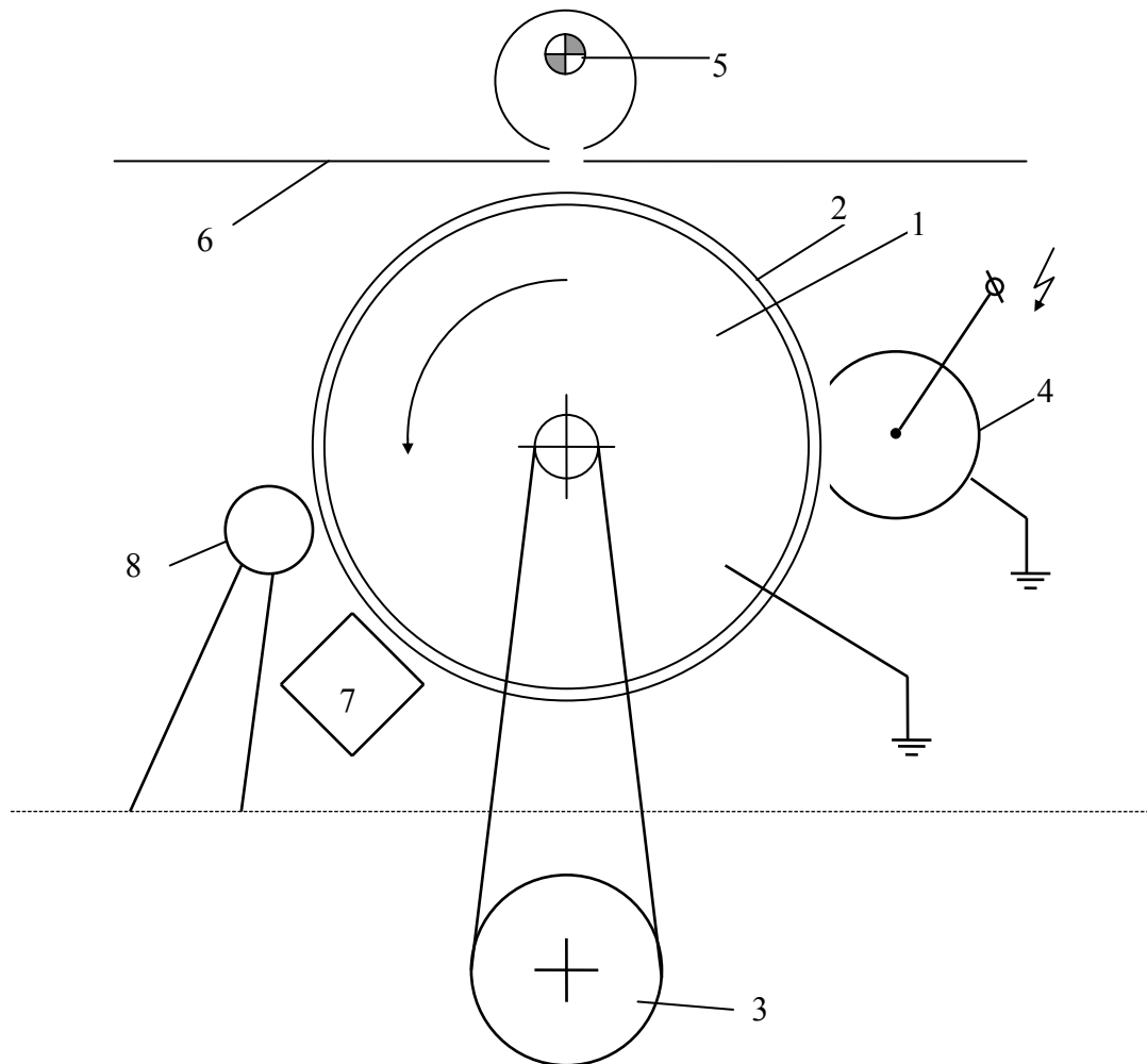
Рис. 8.2. Схема лабораторного макета электрографического аппарата
